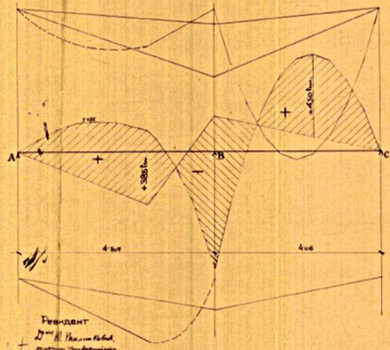
Скица за прорачун статике подрума зграде РВ и ПВО
